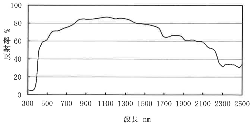
図1 分光反射率
