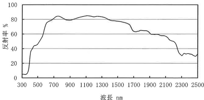
図 1 分光反射率
