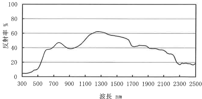
図1 分光反射率
