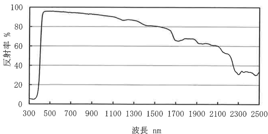
図 1 分光反射率
